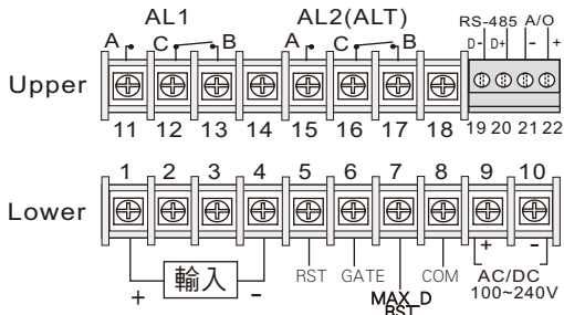
2段瞬間量警報接線方式:
