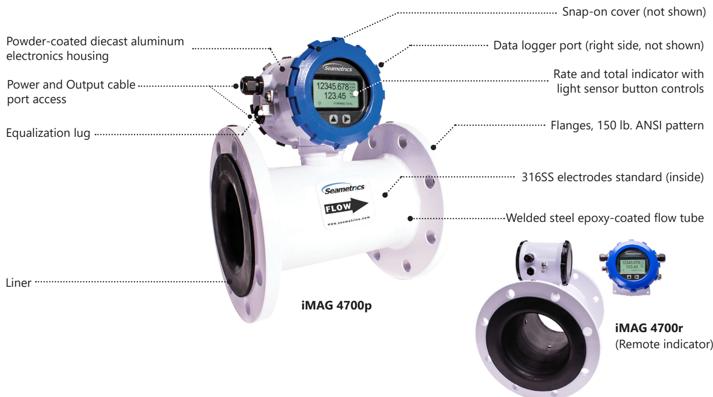
iMAG 4700
