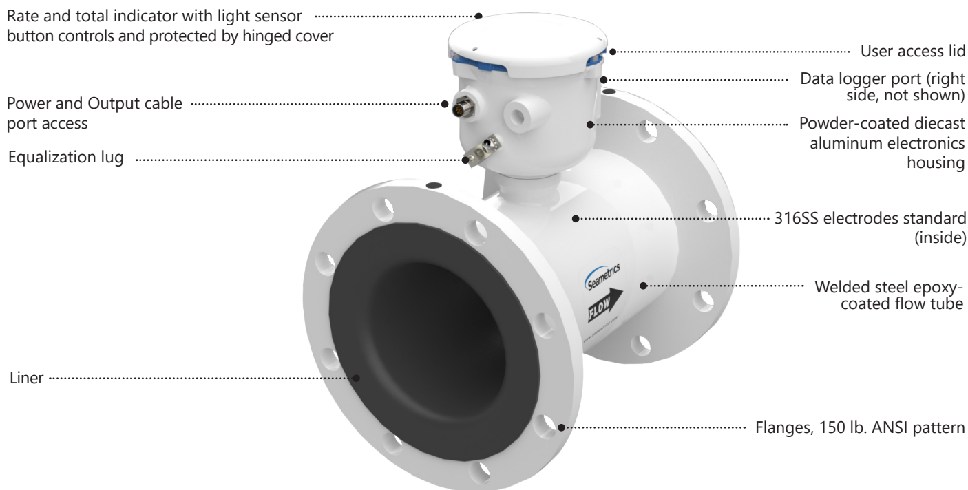
iMAG 4700
